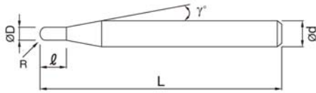
型式 I：全刃長型
